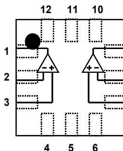
NJM2904CME2 (Note1, 2, 3)
