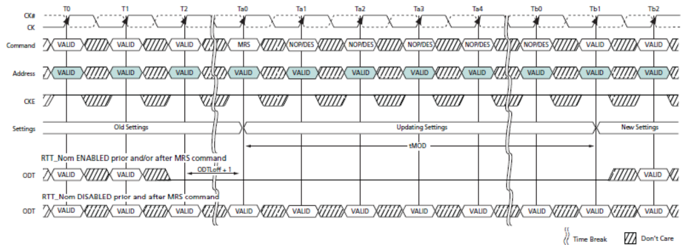
Fig. 4: tMOD Timing
