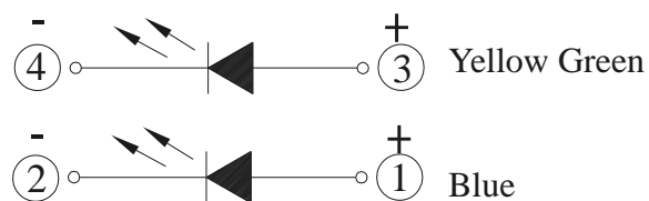
Polarity
