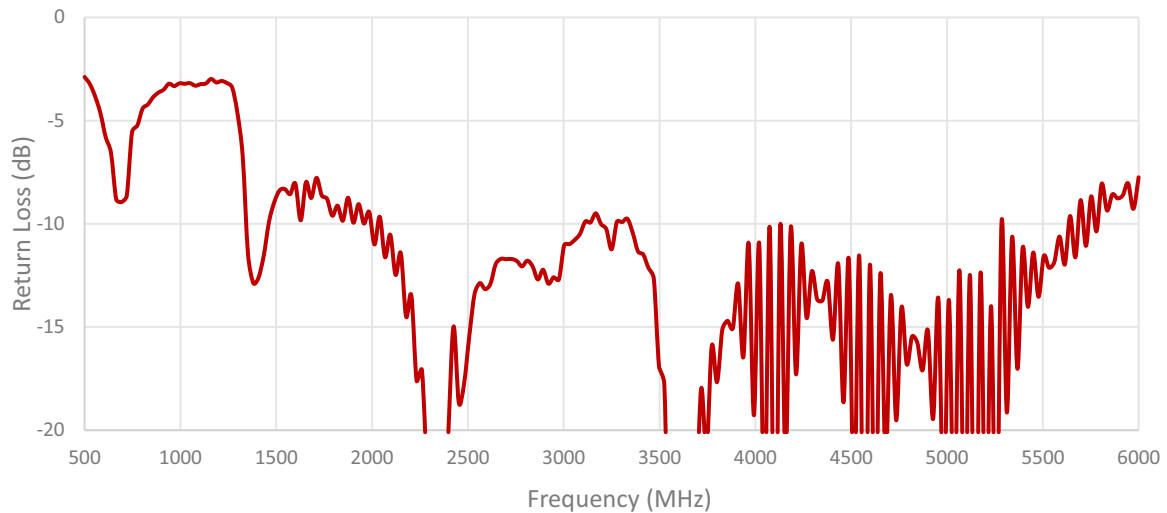
Cable 3: 5GNR
