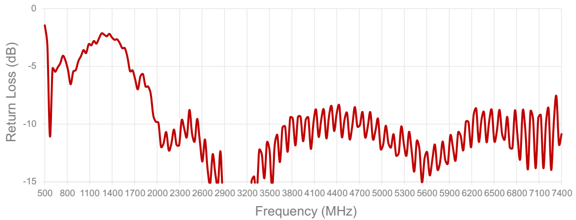
Cable 1: 5GNR
