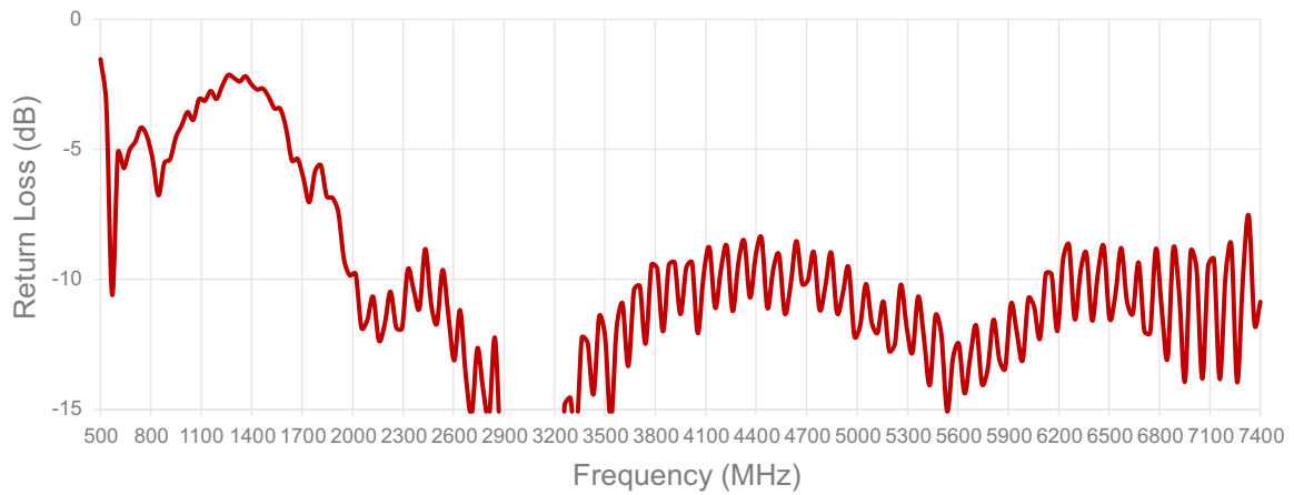
Cable 2: 5GNR
