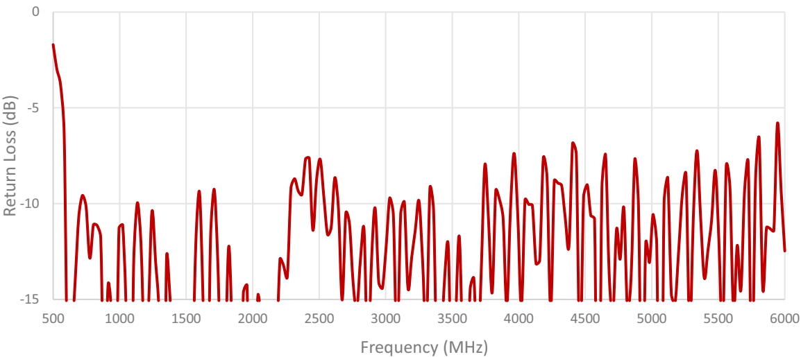
Cable 1: 5GNR
