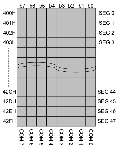
48 SEG x 8 COM LCD Memory Map
