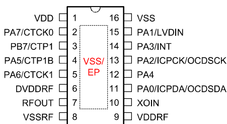
BC68F3132/BC68V3132 16 NSOP-EP-A
