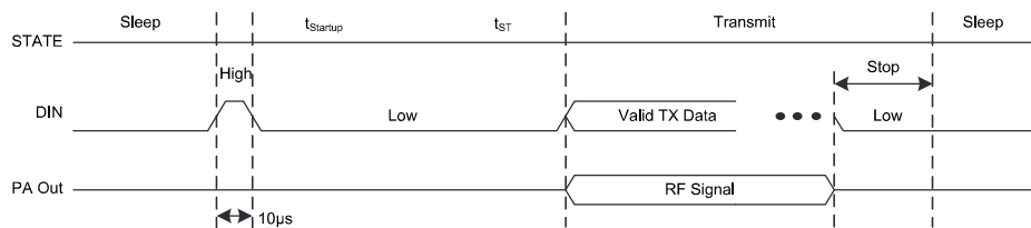
TX Enabled by DIN Input
