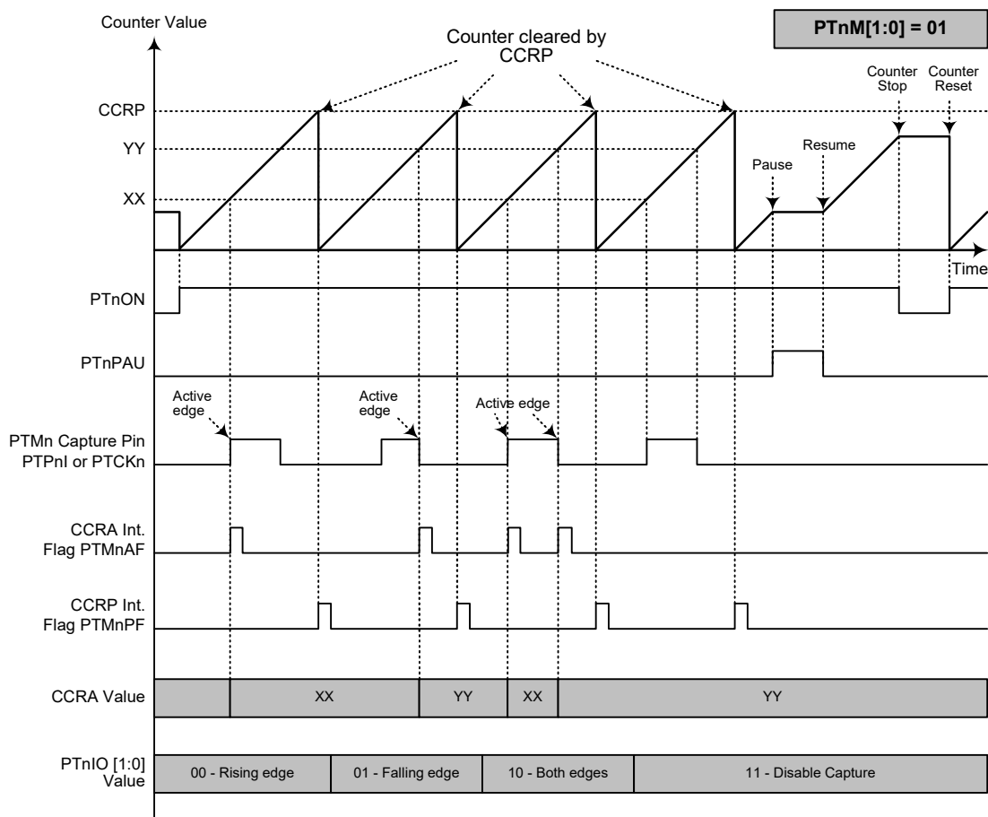
Capture Input Mode (n=1~2)
